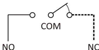
Rysunek 3-2 Struktura obwodu wyjściowego przekaźnika
